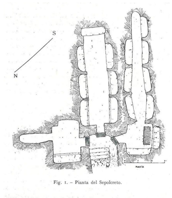
Pianta del sepolcreto. Il vestibolo si apre verso nord-ovest; tre porticine immettono nei tre ambienti. Disegno N. Antonioni, Soprintendenza di Roma II (Morpurgo 1944-45, fig. 1).
